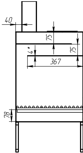
А-А (1 : 15)
