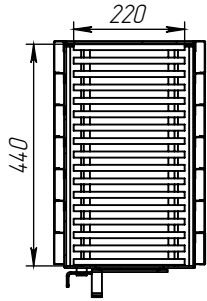
В-В (1 : 15)
